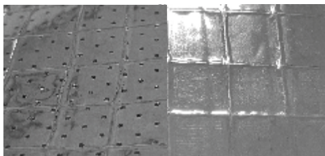
PELLICOLE MICROFORATE, PELLICOLE NON MICROFORATE La prima è permeabile al vapore e la seconda è impermeabile al vapore per una buona regolazione dell'umidità nel sottotetto.
