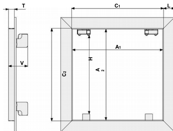
Misure installazione | Foro luce | Altezza
